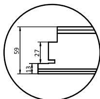
Rez dverí
