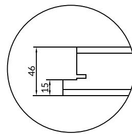
Rez dverí (grubość 46mm)
